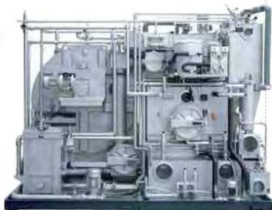
Parte posterior
